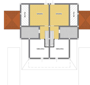
Planimetria Piano primo
